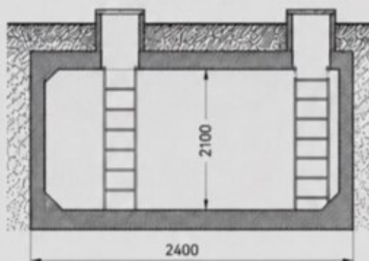
РАЗРЕЗ (вид сбоку)
